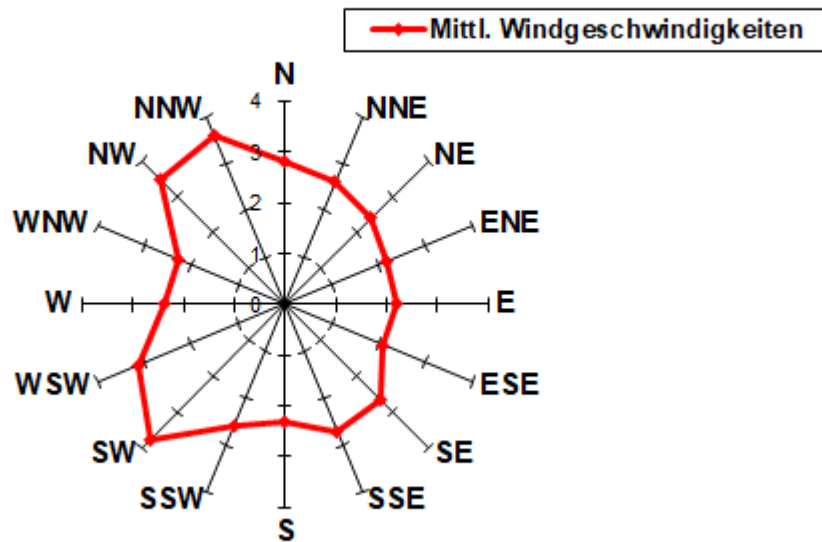
Mittl. Windgeschwindigkeiten pro Windrichtung Hohenheim, April 2023
