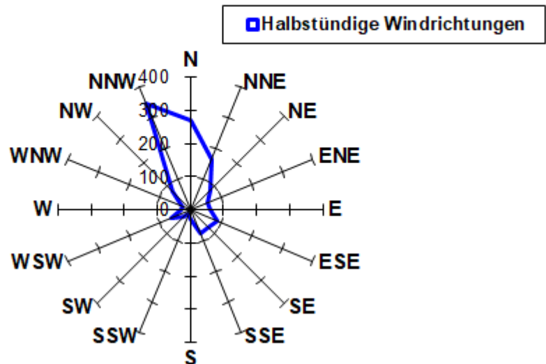
Häufigkeit der verschiedenen Windrichtungen / Hohenheim, Mai 2023
