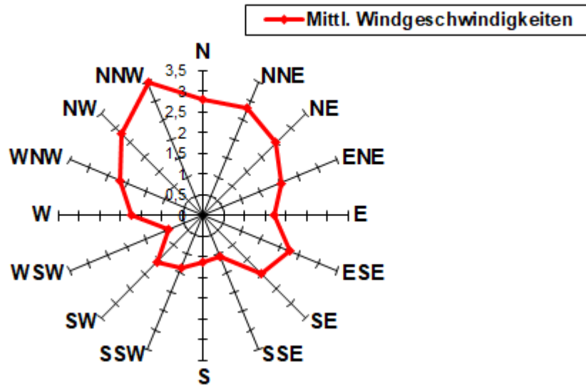
Mittl. Windgeschwindigkeiten pro Windrichtung Hohenheim, Mai 2023
