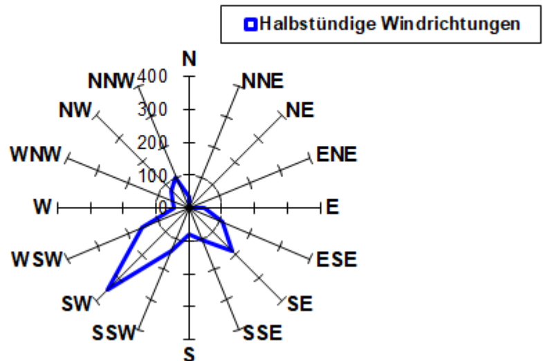
Häufigkeit der verschiedenen Windrichtungen / Hohenheim, Oktober 2023
