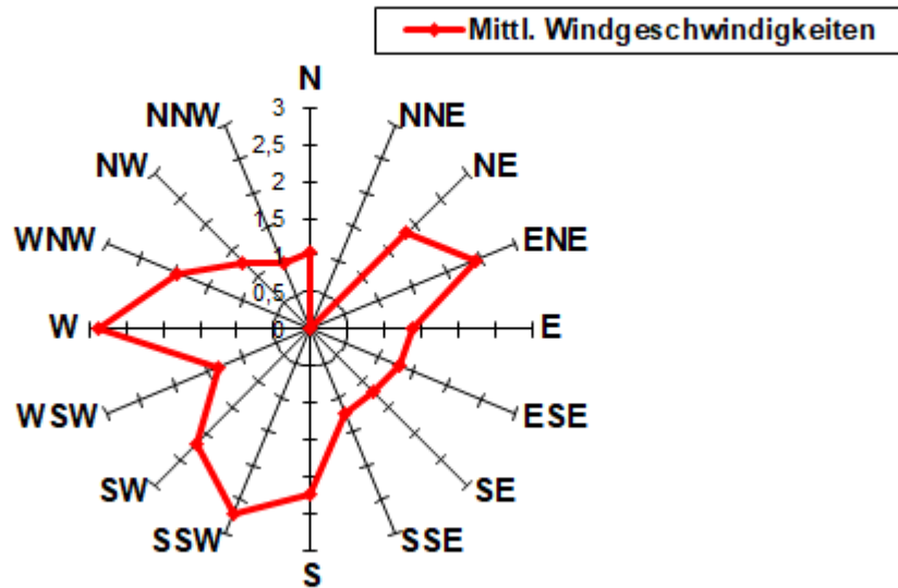
Mittlere Windgeschwindigkeiten pro Windrichtung Hohenheim, Oktober 2023
